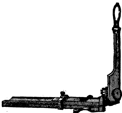
Рѣзакъ для шпонѣ.
